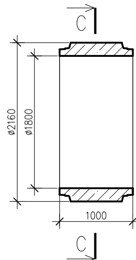
PRZEKRÓJ D-D
